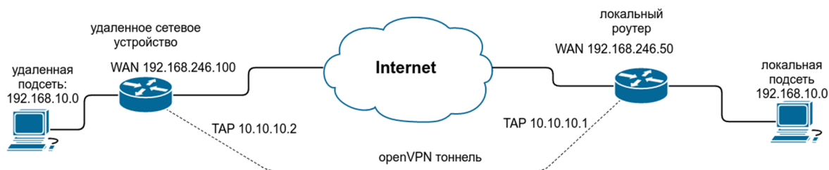
Рис. 3 Примеры конфигураций OpenVPN. Схема сети
