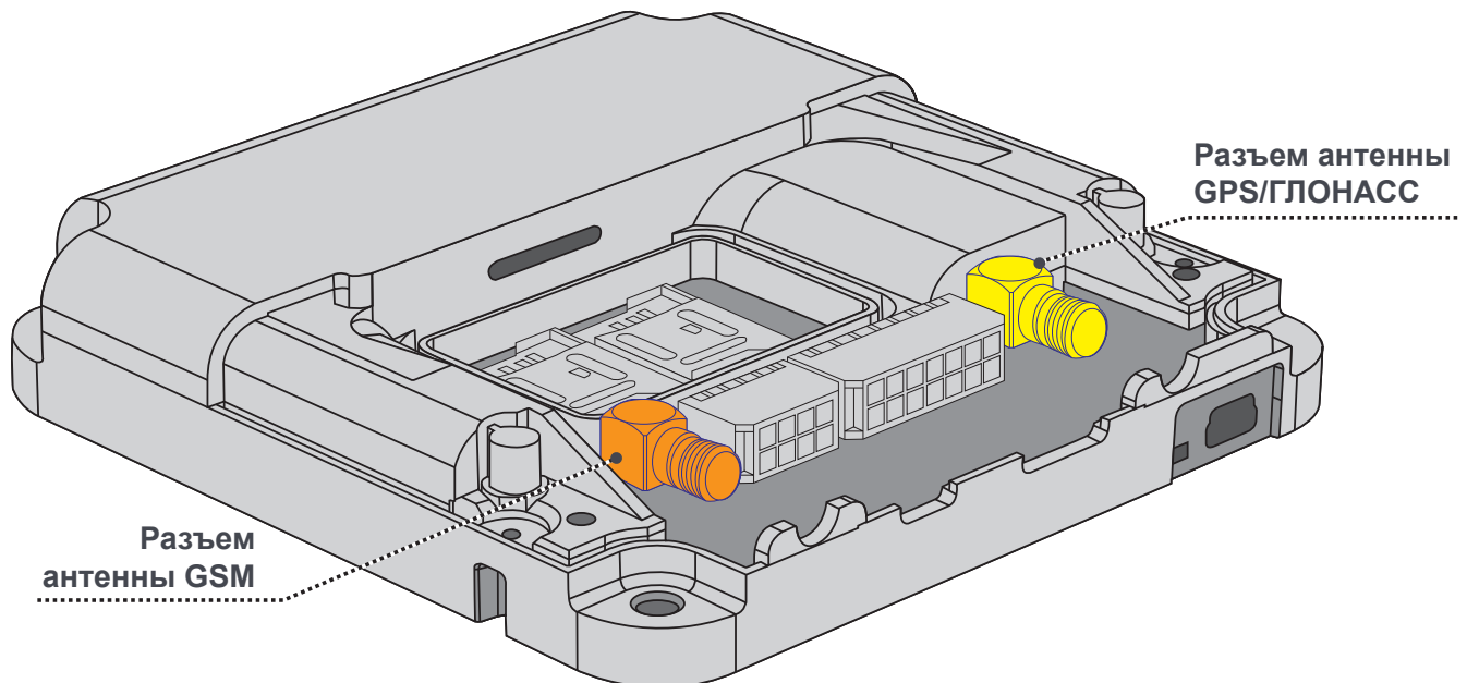
Рис. 2.6. Положения разъемов антенн в навигационном терминале iON Pro
