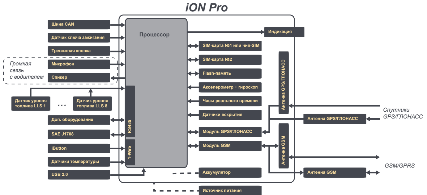
Рис. 1.4. Структурная схема навигационного терминала iON Pro
