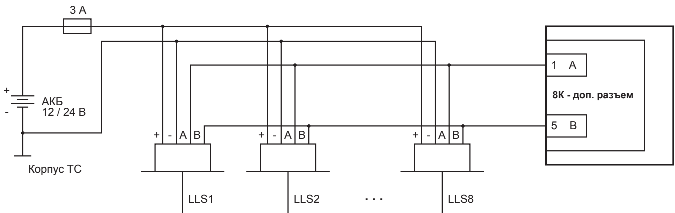
Рис. 3.4. Схема подключения датчиков LLS (ДУТ) через RS485 (1)
