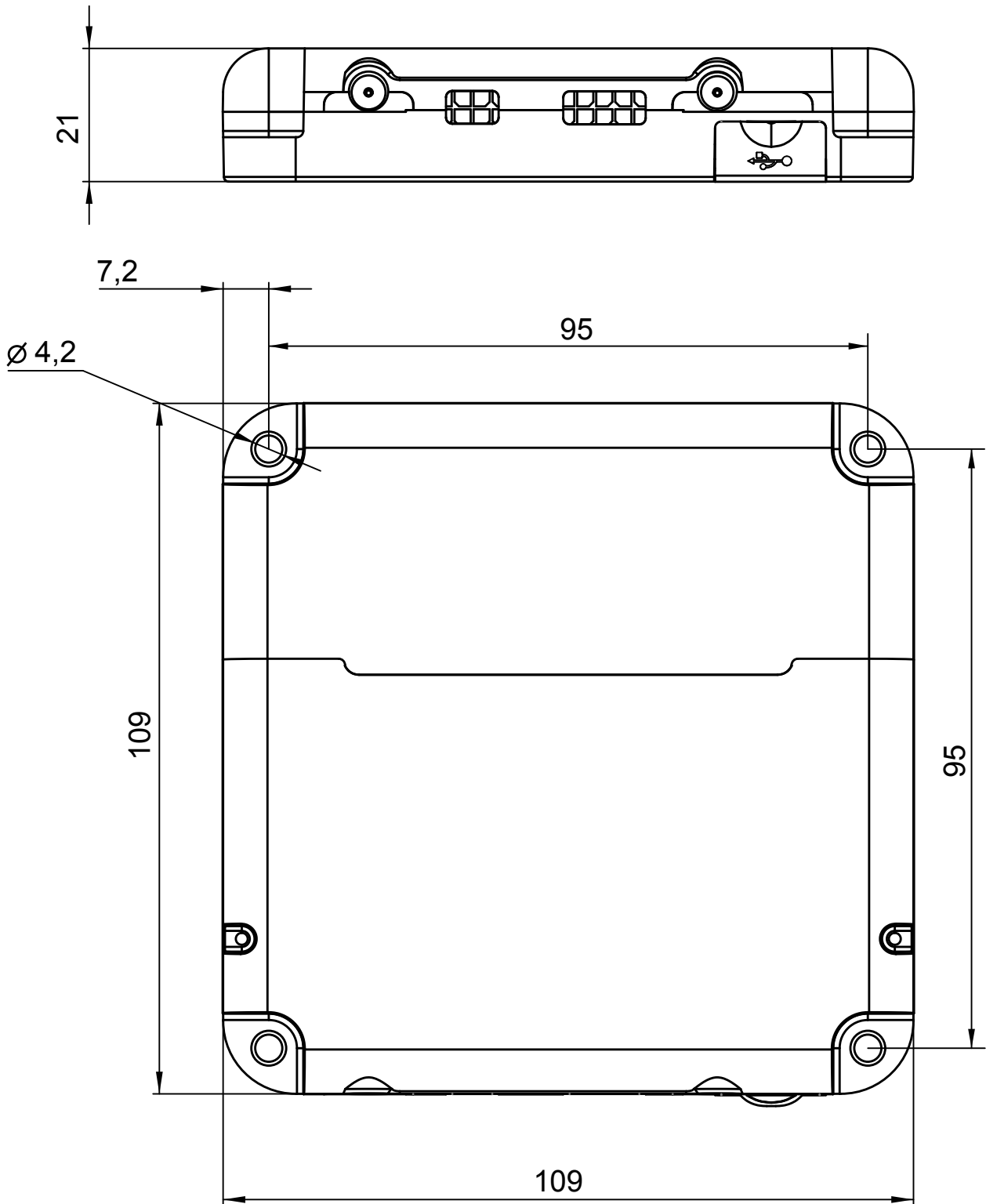
Рис. 1.6. Габаритный чертеж навигационного терминала iON Pro
